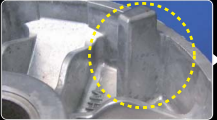
正常なプリーリブ
