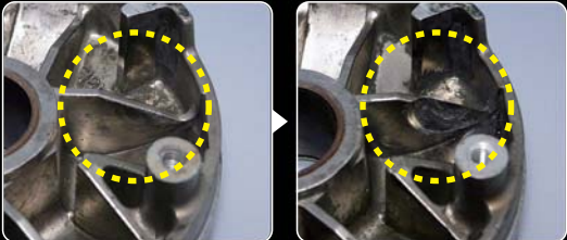
正常な状態のローラーガイド 破損した状態のローラーガイド
