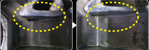
正常にウエイトローラーが装着されていたガイド部分。 磨耗しガイド部分が薄くなっている
